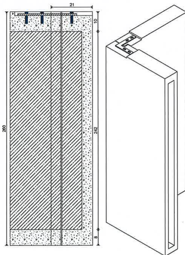
Figure 12 b : Panneaux sandwichs d'habillage d'ossature (type bâtiment avicole) – coupe en élévation sur jonction d'angle
