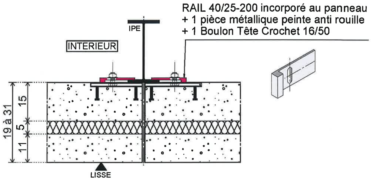
Figure 15 : Panneaux sandwichs d'habillage d'ossature (type longrine de bâtiments industriels) – coupe horizontale – fixation par crapaud
