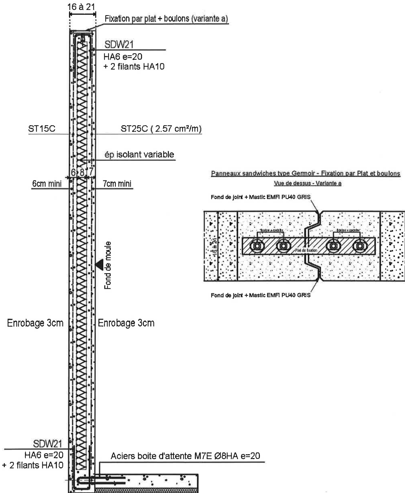
Figure 7 : Panneaux sandwichs de façade posés sur plots (type gerموir) – variante a- coupe verticale
