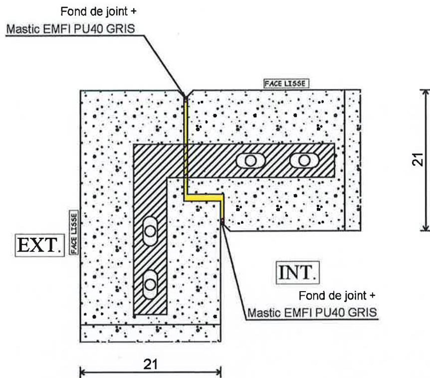
Figure 12 a : Panneaux sandwichs d'habillage d'ossature (type bâtiment avicole) – coupe horizontale - détail sur jonction d'angle
