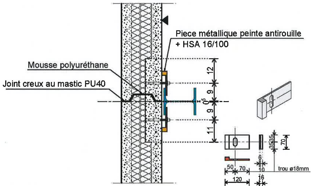
Figure 13 : Panneaux sandwichs d'habillage d'ossature (type longrine bâtiment avicole) – coupes verticales et horizontales variante a
