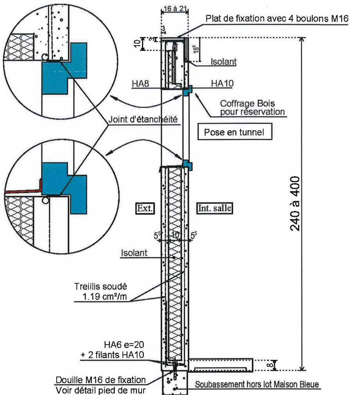
Figure 3 : Panneaux sandwichs de façade posés sur soubassement- Type bâtiment d'élevage porcin - coupe verticale – avec réservation en coffrage en bois
