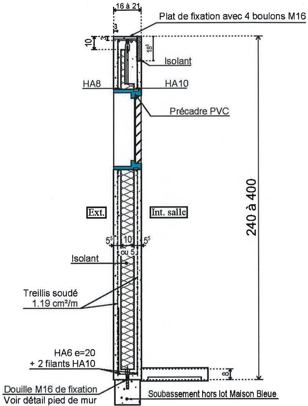
Figure 2 : Panneaux sandwichs de façade posés sur soubassement – Type Bâtiment d'élevage porcin- coupe verticale – avec précadre PVC
