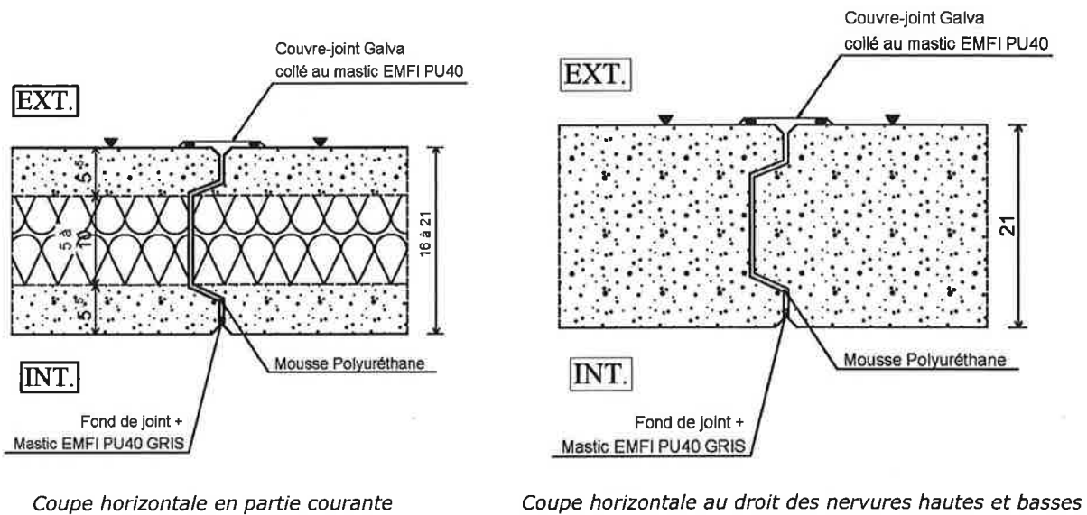
Figure 5 : Panneaux sandwichs de façade posés sur soubassement – traitement de joint vertical
