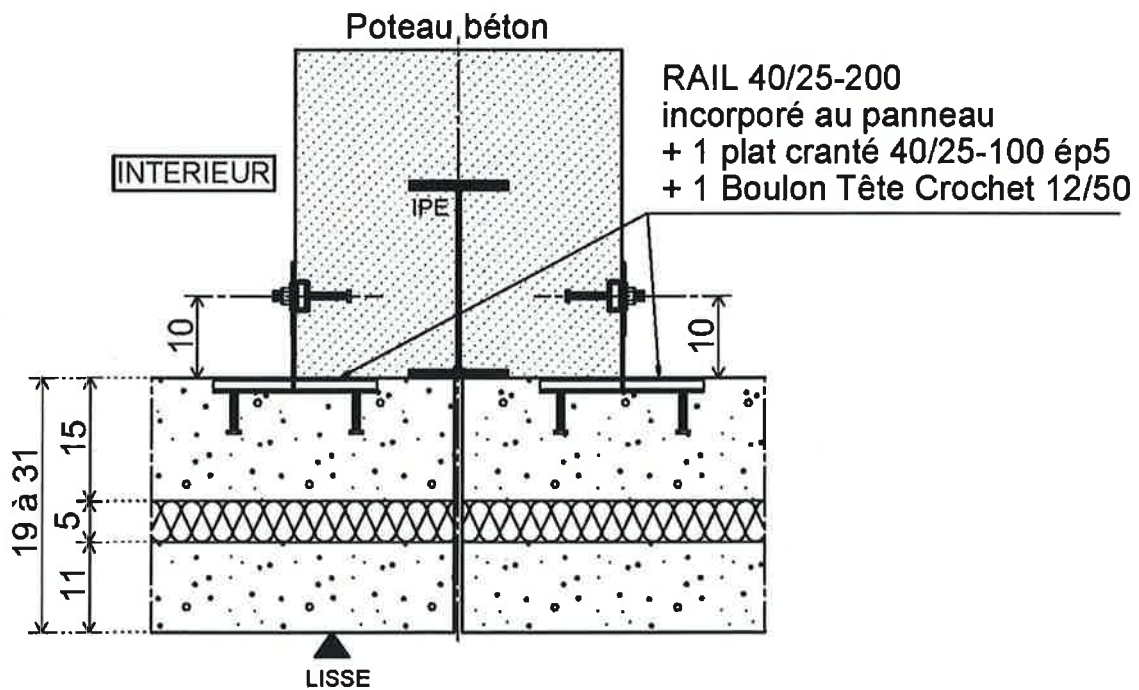
Figure 16 : Panneaux sandwichs d'habillage d'ossature (type longrine de bâtiment industriel) – coupe horizontale – fixation par rail
