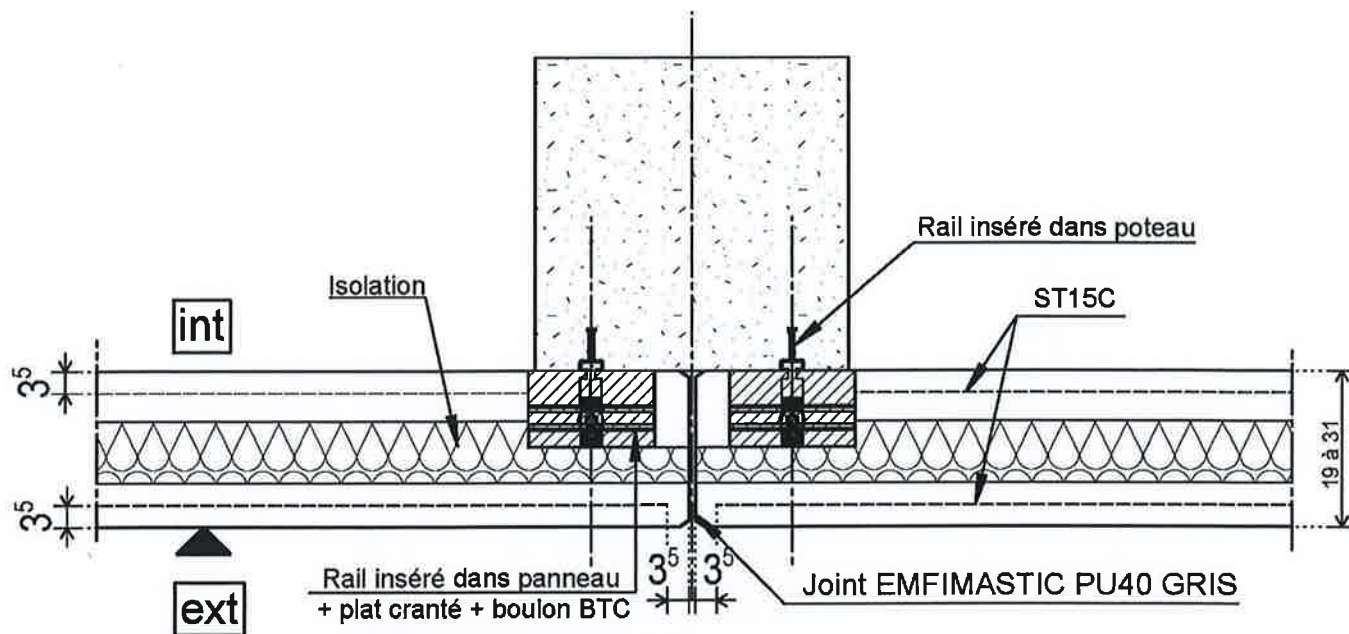
Figure 22 : Panneaux sandwiches-fixation sur poteau béton - coupe horizontale
