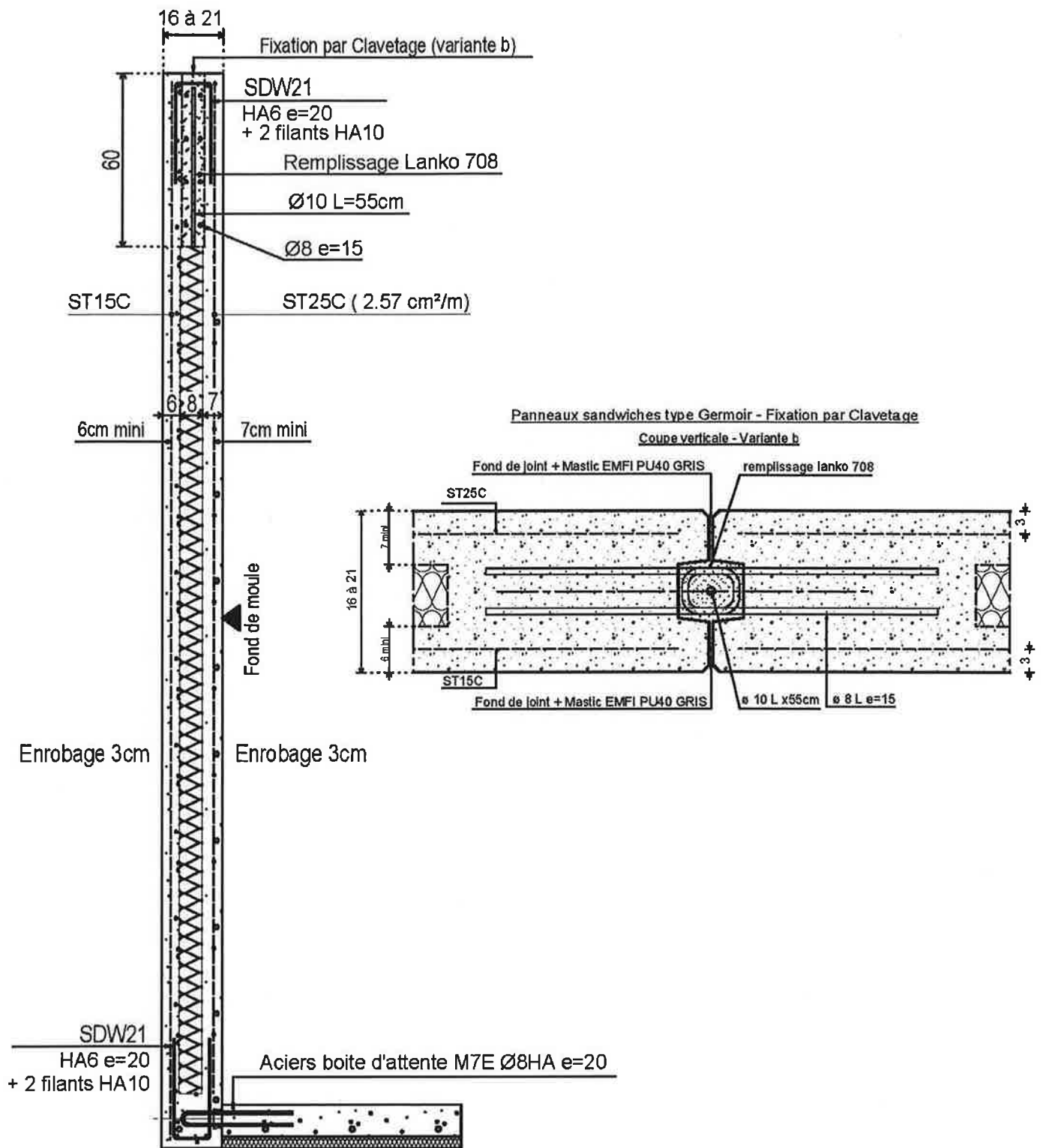
Figure 8 : Panneaux sandwichs de façade posés sur plots (type germoir) – variante b– coupe verticale
