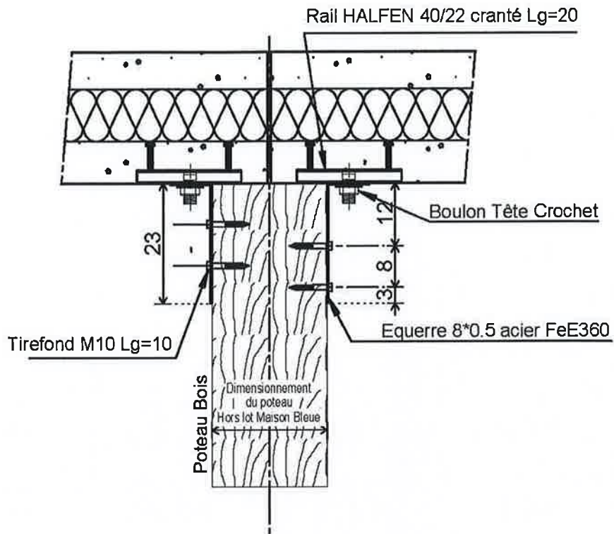
Figure 24 : Panneaux sandwiches- Exemple de fixation sur poteau bois en zone sismique – Coupe horizontale
