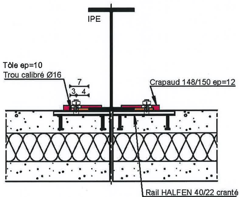
Figure 23 : Panneaux sandwiches- Exemple de fixation sur poteau métallique en zone sismique - coupe horizontale
