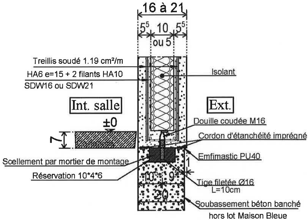
Figure 4 : Panneaux sandwichs de façade posés sur soubassement – détail pied de mur
